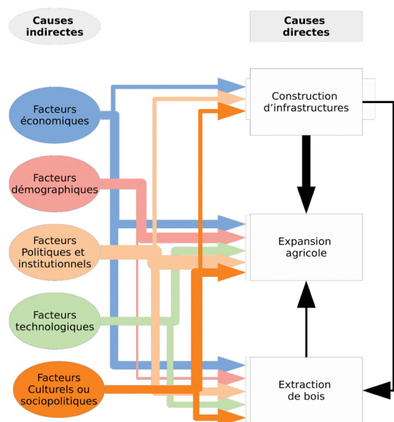
FIGURE 1 - ADAPTÉE DE GEIST ET LAMBIN 2002. LES CAUSES DIRECTES DE DÉFORESTATION (RECTANGLES) S'INFLUENT ENTRE ELLES (FLÈCHES NOIRES) ET SONT INFLUENCÉES (FLÈCHES DE COULEUR) PAR DES CAUSES INDIRECTES (OVALES). LA TAILLE DES FLÈCHES INDIQUE L'IMPORTANCE RELATIVE DES INFLUENCES D'APRÈS L'ÉTUDE DE 152 ÉTUDES DE CAS.
