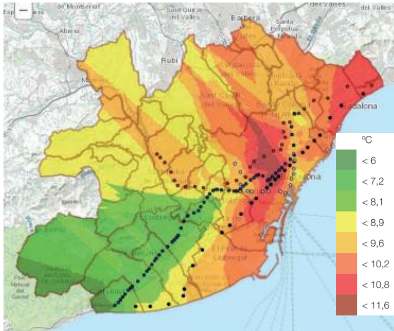
Configuració de l'illa de calor a Barcelona i la seva àrea metropolitana
